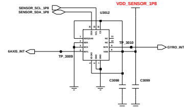
6 AXIS(ACC+GRYO)
