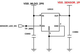
VDD_MLDO_2P0
