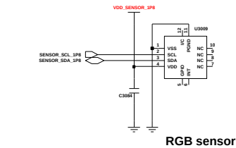
RGB sensor
